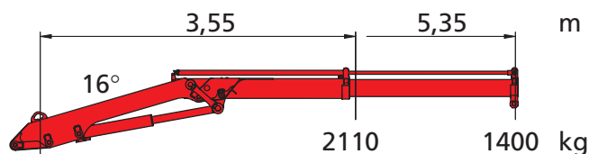
a1 5,42 m max. hydraulische Reichweite (Arm gestreckt) / max. outreach (horizontal position)
