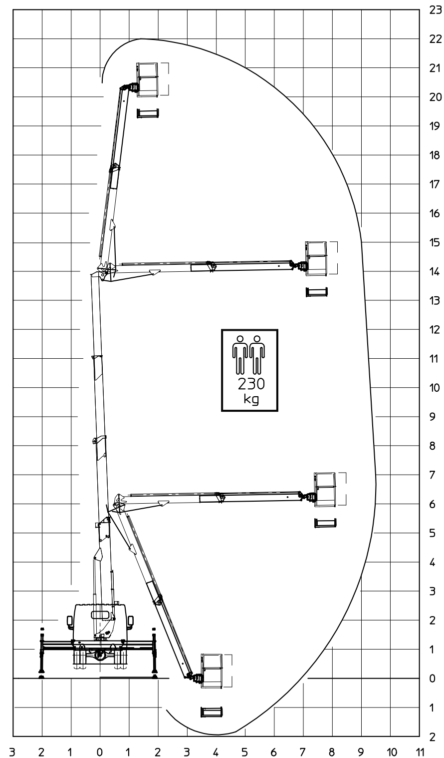
TRAVERSE ESTESE - OUTRIGGER OUT
