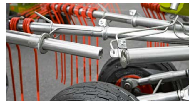
Manchons raccords citron et sécurité PROFIX sur le LINER 700.
