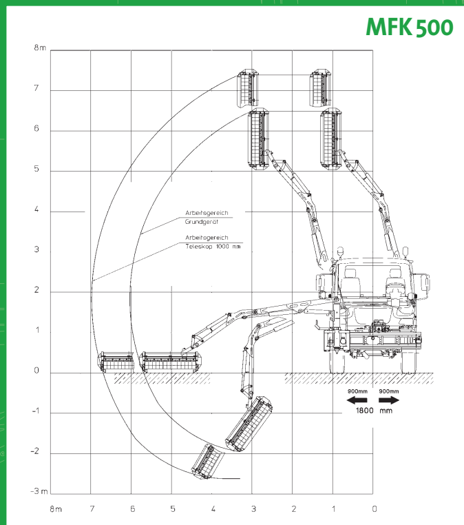
Diagramme de portée MFK 500
