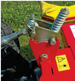
Federbelastete Anfahrtsicherung
