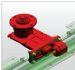
Montagefreundlicher Balkenaufbau
