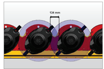
Großer, weit vorn liegender Überschnitt der Mähscheiben
