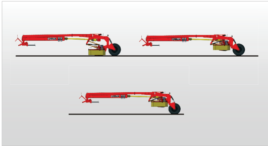
Hoher Aushubweg durch Hydraulikzylinder
