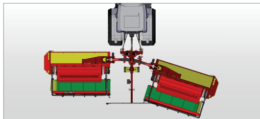
Ausweichen nach hinten
