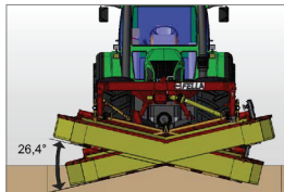
Großer Pendelweg
