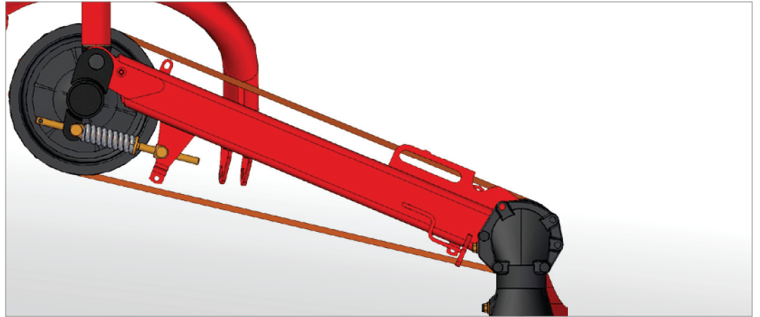
Elastischer Keilriemenantrieb
