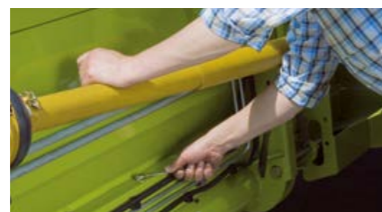
Abstreifer von außen einstellbar (C 490, C 430, C 370).
