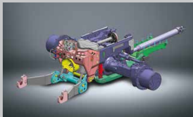
Suspension électronique intégrant un système « anti-plongée » et « anti-cabrage ». La suspension peut servir tant dans les champs que sur route. Entièrement verrouillable au besoin.
